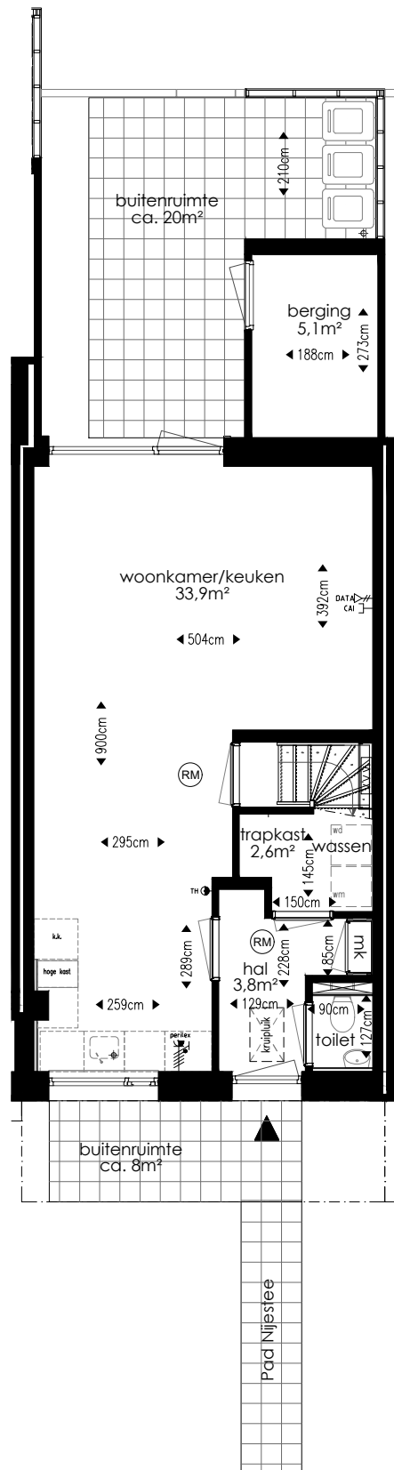
Begane grond
